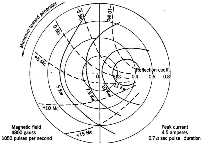
FIG. 19-40.—Rieke diagram for 2J42 magnetron.
